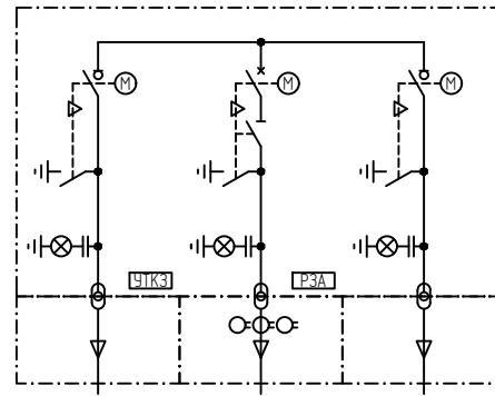
РУ-10 кВ
